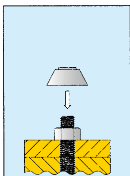
②シャーキャップをかぶせる。
