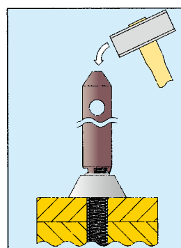
③セッティングツールを使用して ハンマーで叩く。
